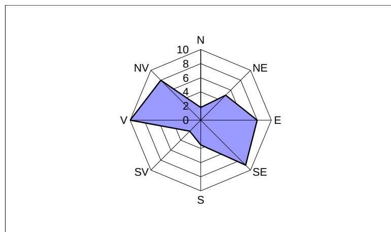
Figura nr. 2.3. Roza direcțiilor vântului la Baia Mare (după Atlasul Republicii Socialiste România 1972- 1979)
