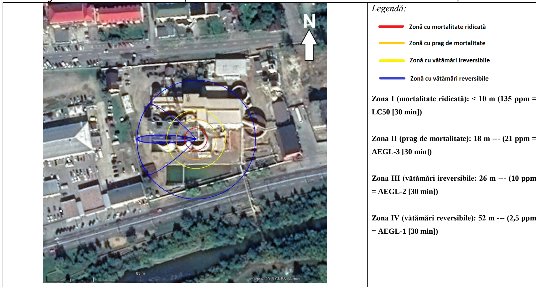
Figura nr. 4.9. Contururi de concentrații de acid cianhidric în cazul emisiei accidentale din tancul CIL1 – condiții meteo medii
