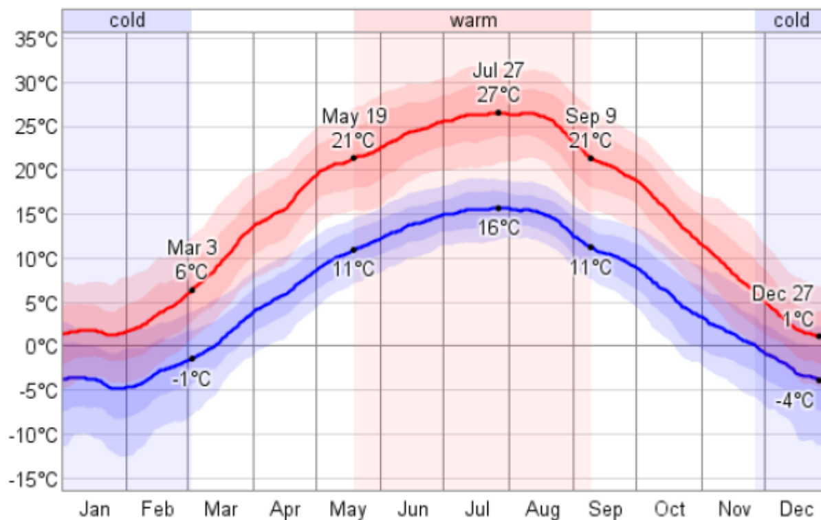
Figura nr. 2.1. Variația valorilor zilnice minime (cu albastru) și maxime (roșu)
