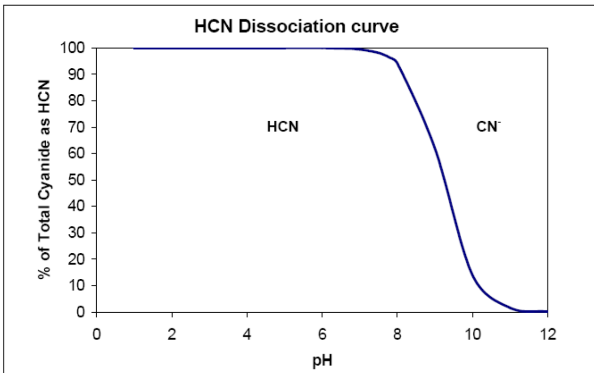
Figura nr. 4.3. Curba de disociere a HCN
